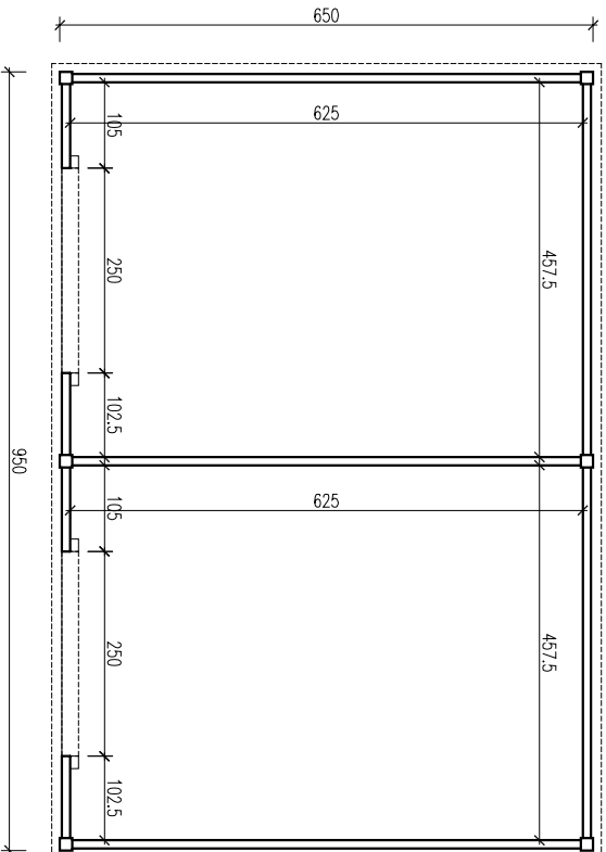
RZUT PARTERU
