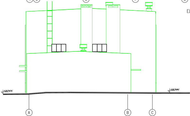
ELEWACJA PÓŁNOCNA
