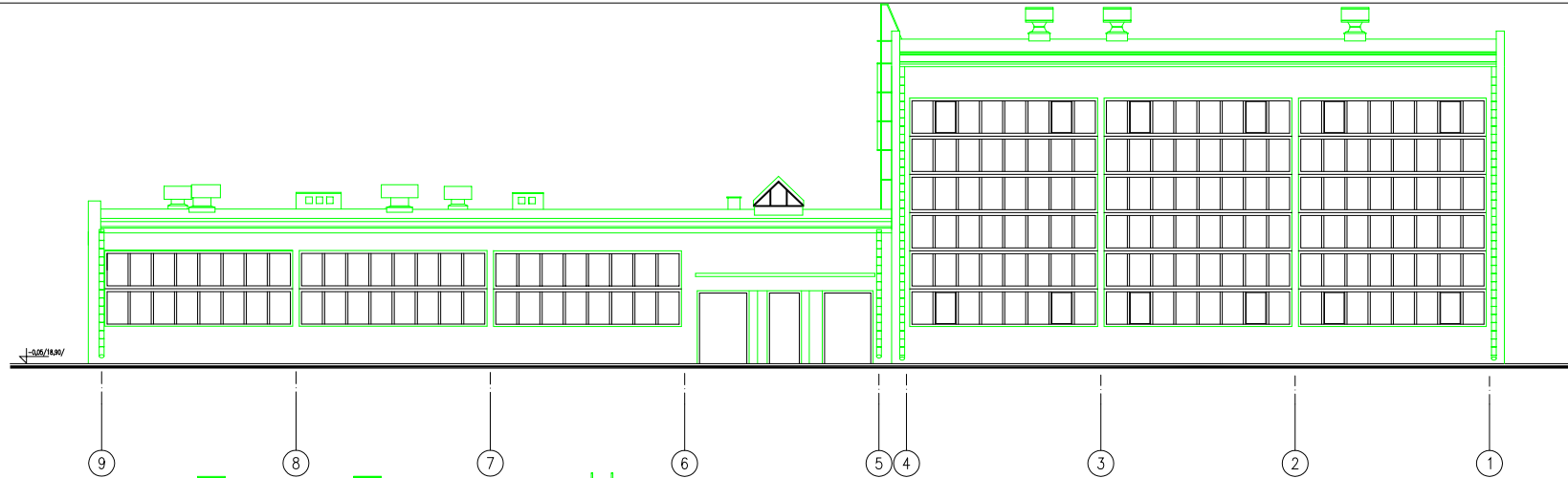
ELEWACJA ZACHODNIA
