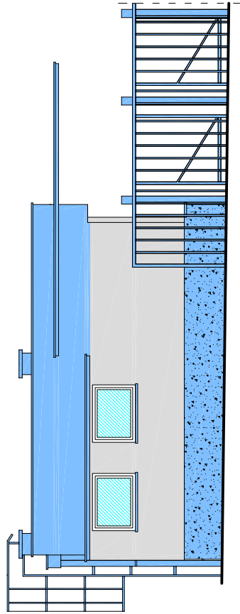
ELEWACJA PÓŁNOCNO–WSCHODNIA
